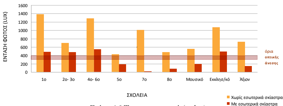
Σχήμα 4.6 Ένταση φωτισμού (σε lux)
