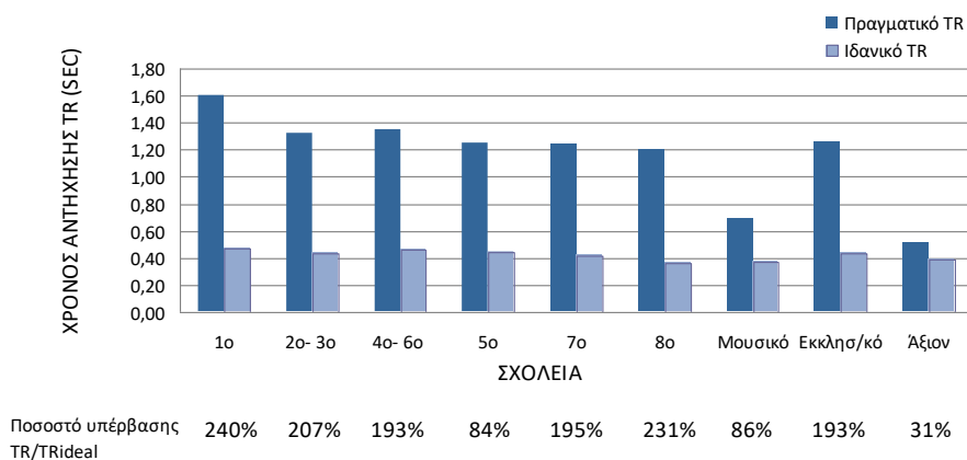
Σχήμα 4.5 Χρόνος αντήχησης αίθουσας στα 500Hz
